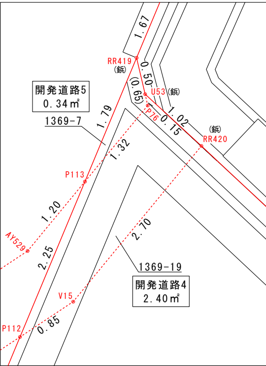
1369-7附近詳細図 1/50
